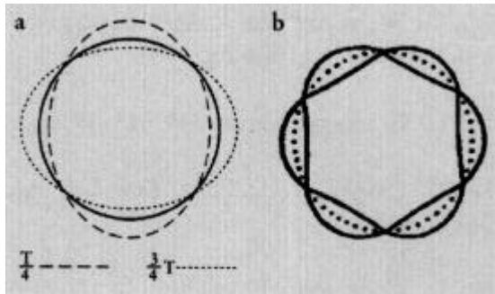
Abb. 2: Schwingungsmoden des Glases (stark übertrieben gezeichnet). (a) Grundschiwingung (b) Oberschiwingung.
