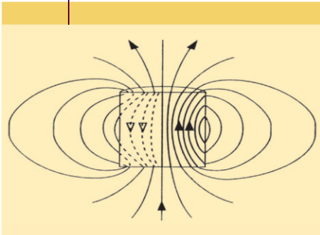
Schnitt durch den Permanentmagneten mit eingezeichneten Magnetfeldlinien.
