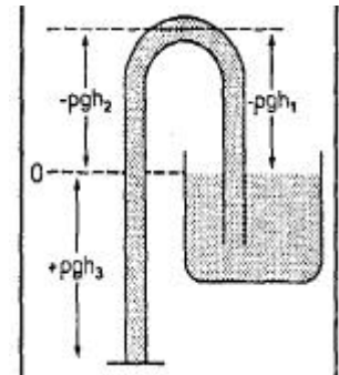
Abb. 6: Wie ein von der Tischkante rutschendes Seil sinkt der Flüssigkeitsfaden
