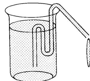
Abb. 5: Konstruktion eines Syphons, der beim Eintauchen in die Flüssigkeit von selbst startet.
