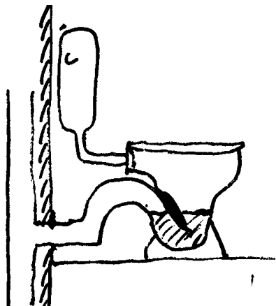
Abb. 4: In dieser Querschnittszeichnung eines WC erkennt man unschwer den als Geruchsverschluß wirkenden Syphon.
